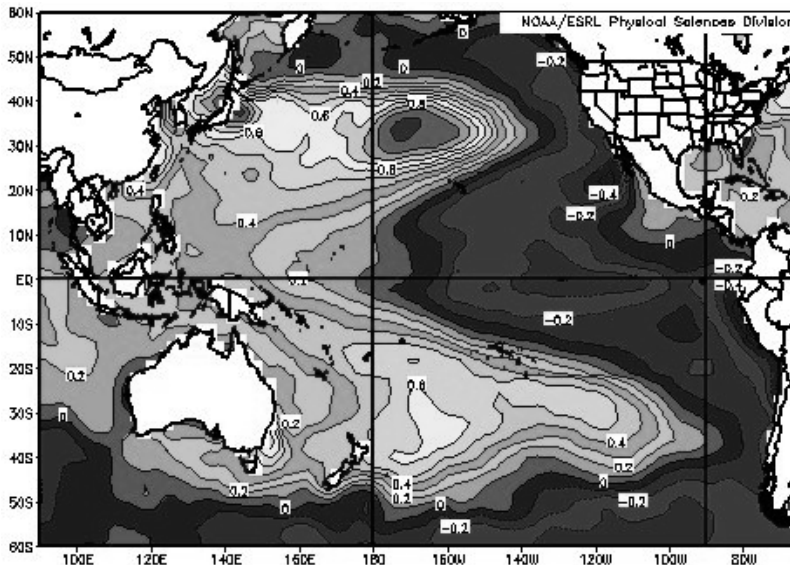
Figura 6. Anomalias da temperatura da superfície do Pacífico no período 1999-2007 (°C), com relação à média do período 1977-1998. (Fonte dos dados: ESRL/PSD/NOAA)
