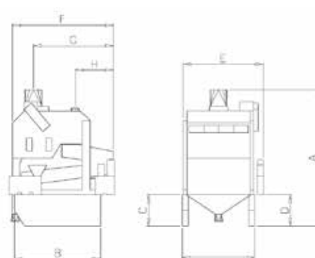
DIMENSÕES GERAIS
