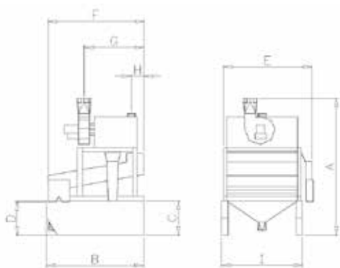
DIMENSÕES GERAIS
