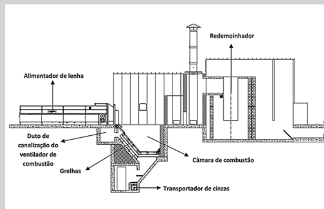
FORNALHA AUTOMÁTICA PARA LENHA
